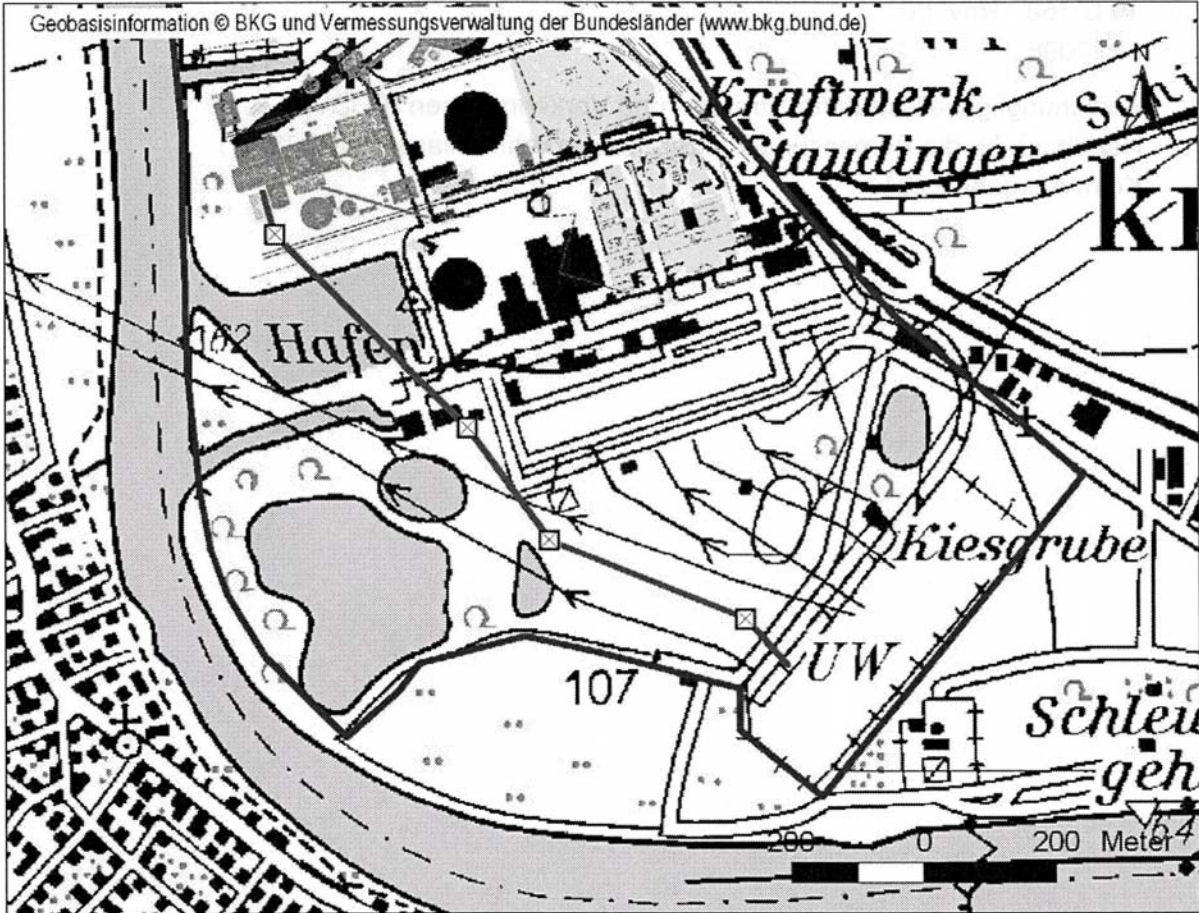
Karte 3: Lage der geplanten 380-KV-Leitung zum Umspannwerk Großkrotzenburg
